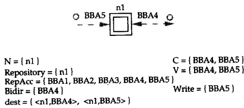
Fig. 10. Interface of Fig. 9.
